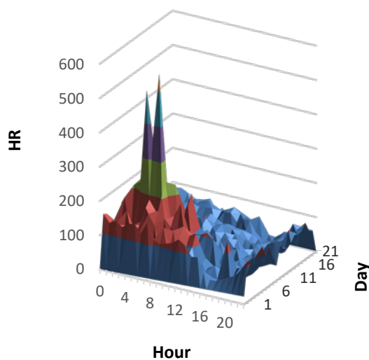
Figura 4. Il grafico mostra l'attività dello sciame nel periodo selezionato. Sull'asse delle ordinate vi è l'ora, su quello delle ordinate il giorno e la quota rappresenta il tasso orario
